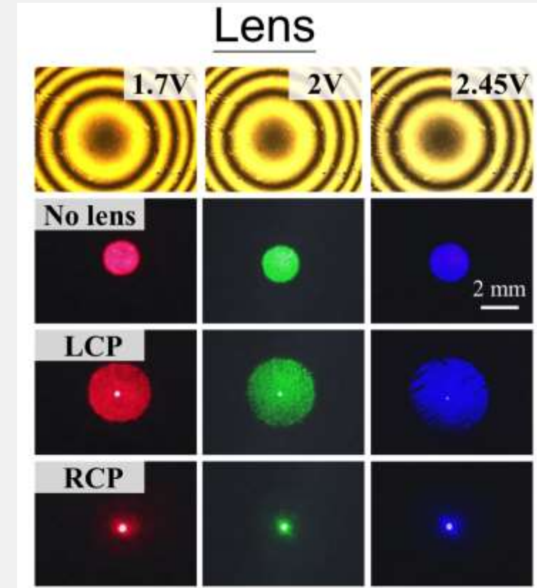
液晶透鏡
